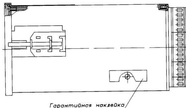
Рисунок 2 – Схема защиты от несанкционированного доступа
